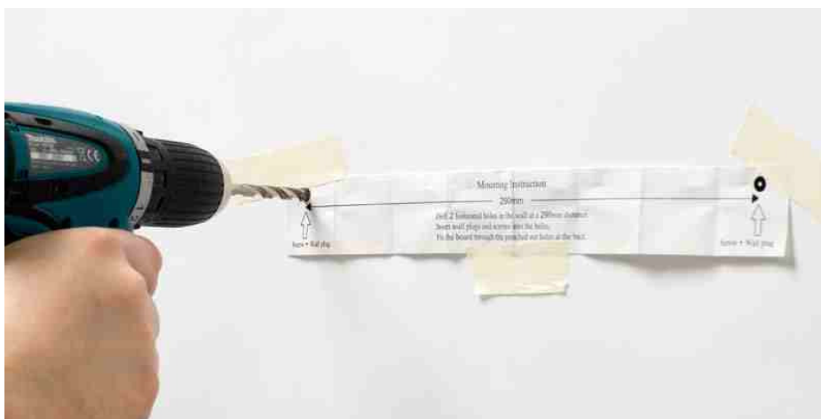
Wiercenie otworów w podłożu przy użyciu szablonu
